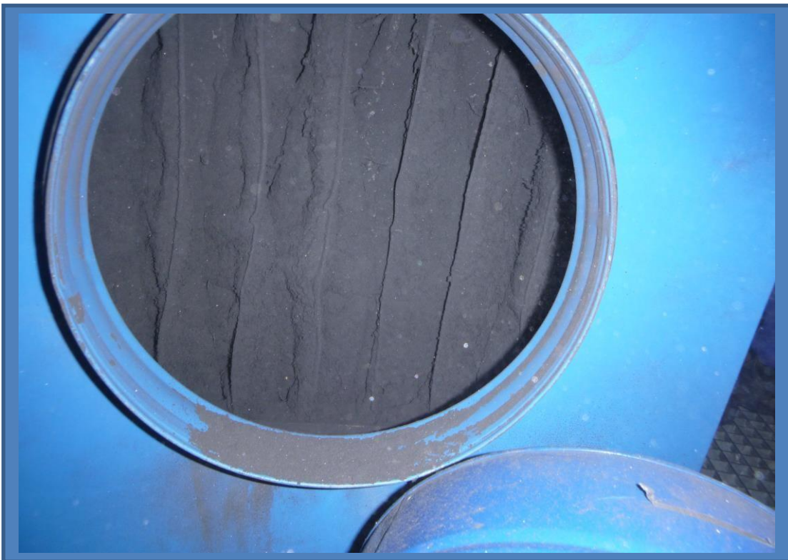
Taschenfilter in der Filterbox 5000m3 (Ursprüngliche Farbe = weiss)
